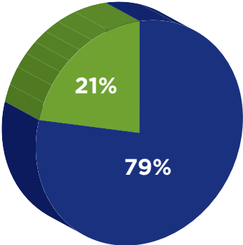
ESOL
